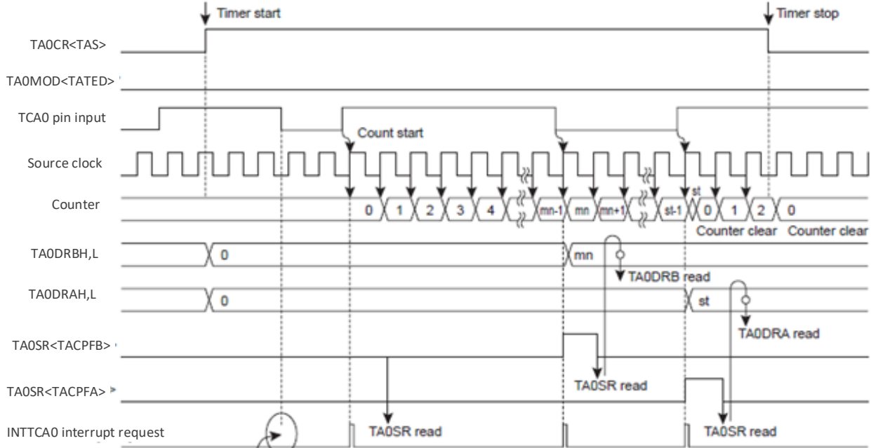
图 13- 19 脉宽测量模式时序图(TCA0 为范例)
