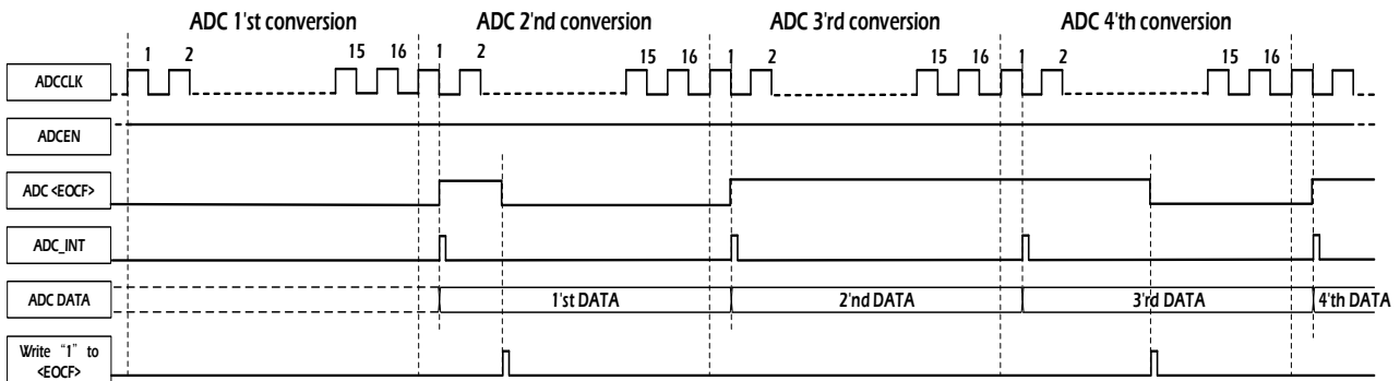
图 8-3 ADC<EOCF>与数据总线时序图
