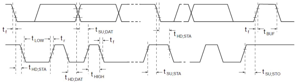
图 15-23 时序定义(No.1)
