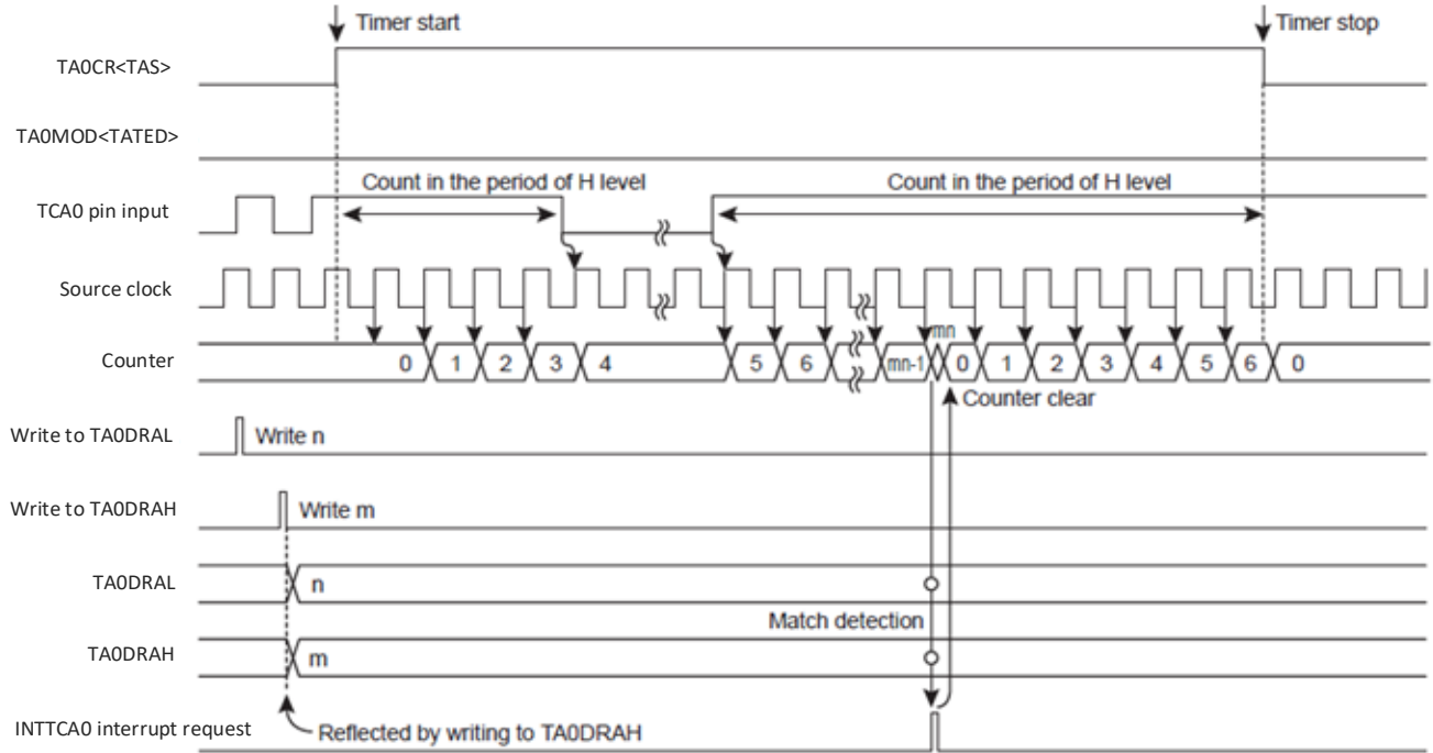
图 13- 18 窗模式时序图(TCA0 为范例)
