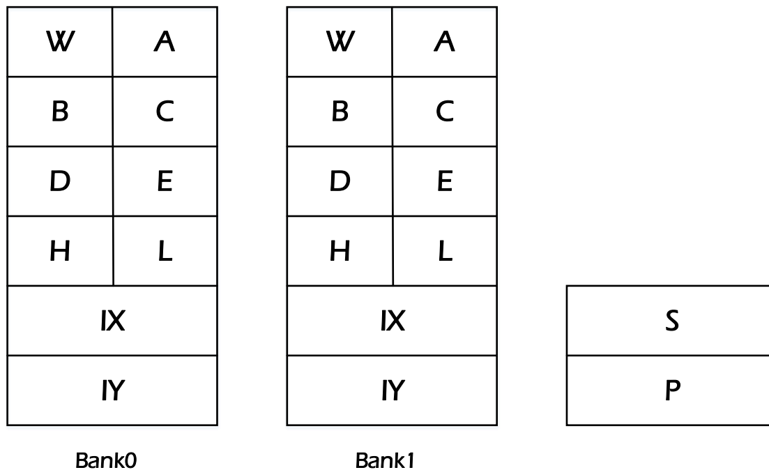
图 4-1 核心寄存器
