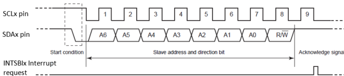
图 15-9 产生开始条件与从属地址
