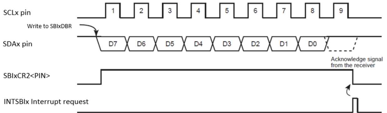
图 15- 18 SBIxCR1<BC>='000'与 SBIxCR1<ACK>='1' 传输
