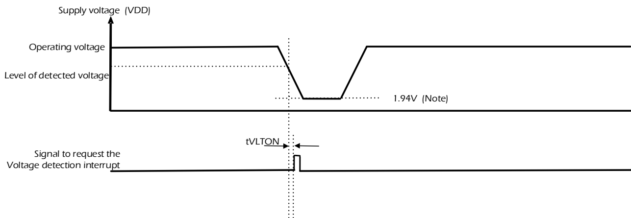
图 3- 3 LVD 中断
